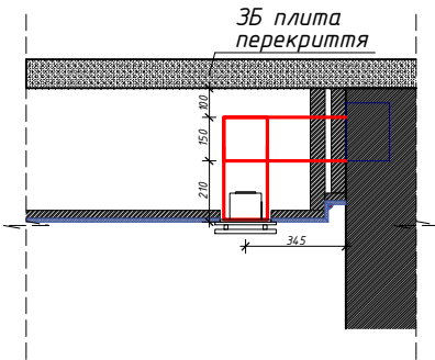
Розріз V2-V2
