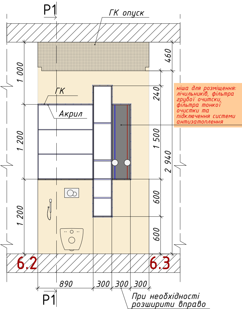
Розгортка 6.2-6.3
