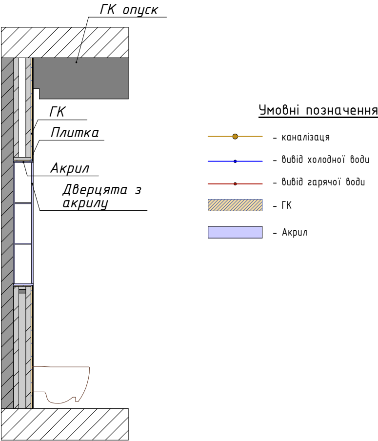
Розріз Р1-Р1
