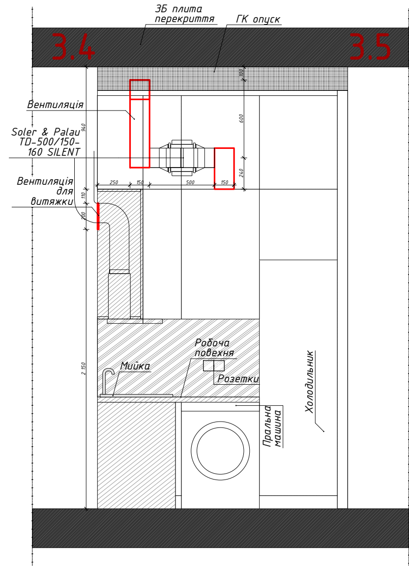
Розгортка 3.4-3.5
