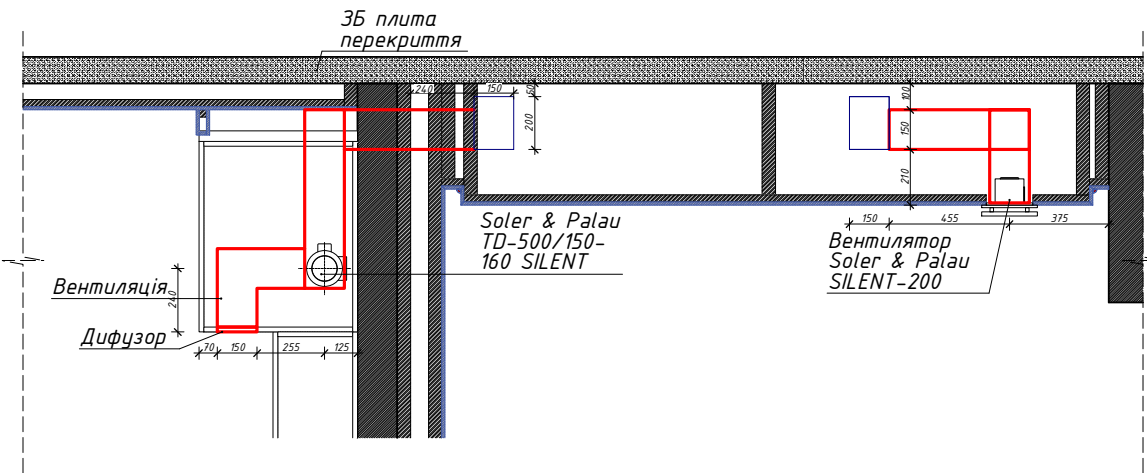
Розріз V1-V1
